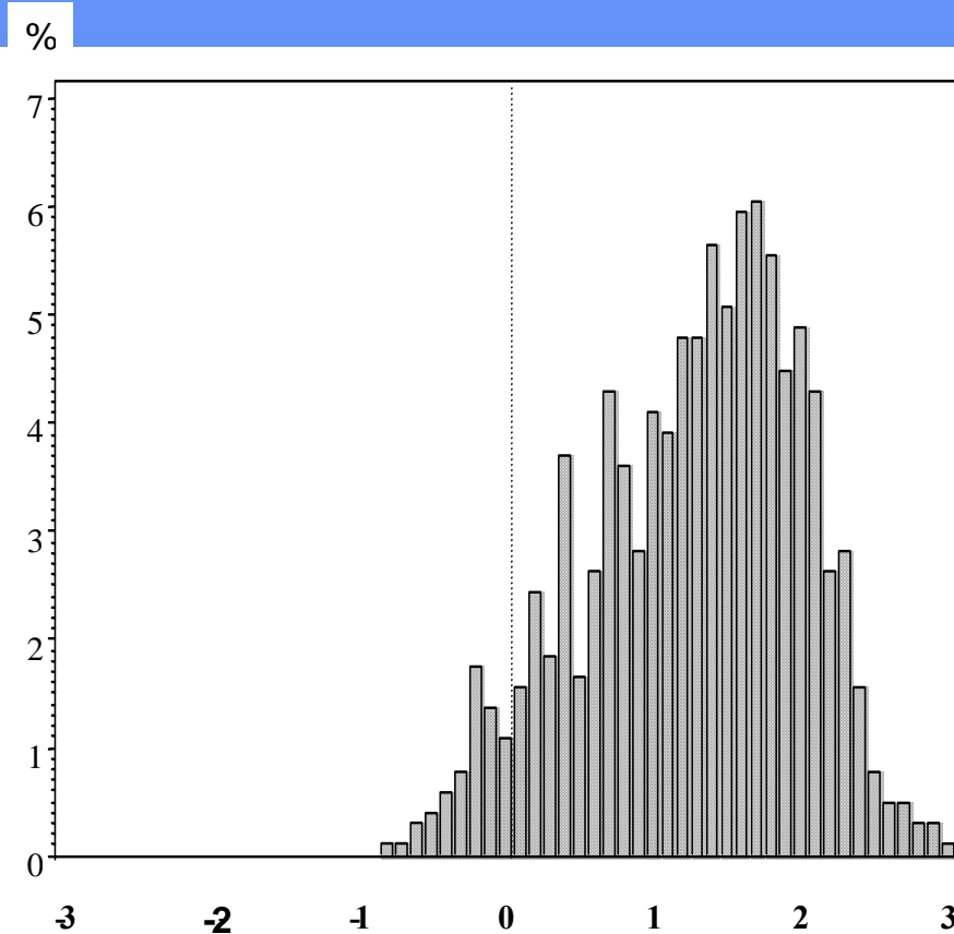
Produit : asymétrique
