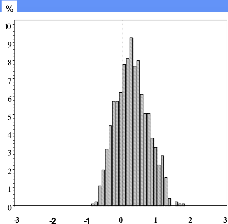
Procédé : symétrique
